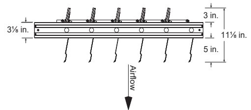
EM-40 No Flange
