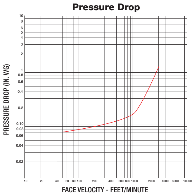
AMCA FIG. 5.7A
