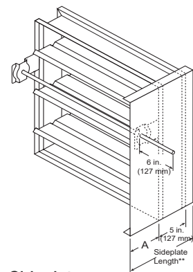
Sideplate
