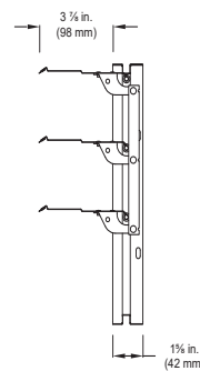
BD-330 No Flange Frame
